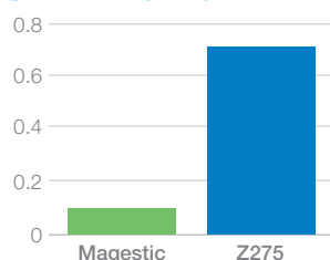
Úbytek materiálu v alkalickém prostředí (pH11,7-5 % čpavku)
