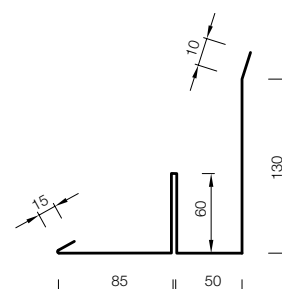
LZN- lem. ke zdi podélné s nosem, r. š. 410 mm
