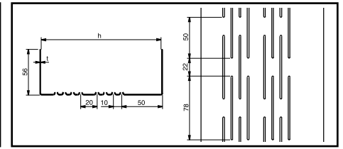
SKY Vnější stěnový vodící profil
