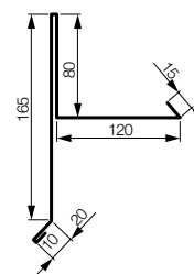
LZN- lem. ke zdi podélné s nosm, r. š. 410 mm
