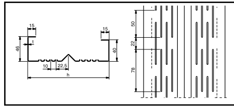
RY Vnější stěnový profil
