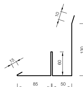
LZN- lem. ke zdi podélné s nosm, r. š. 410 mm
